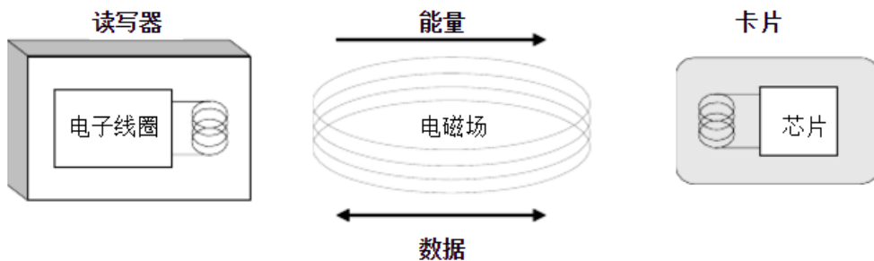
图 射频识别技术原理示意
